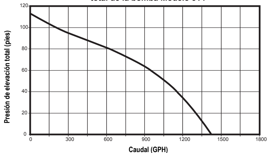
Presión de elevación dinámica total de la bomba Modelo 314
